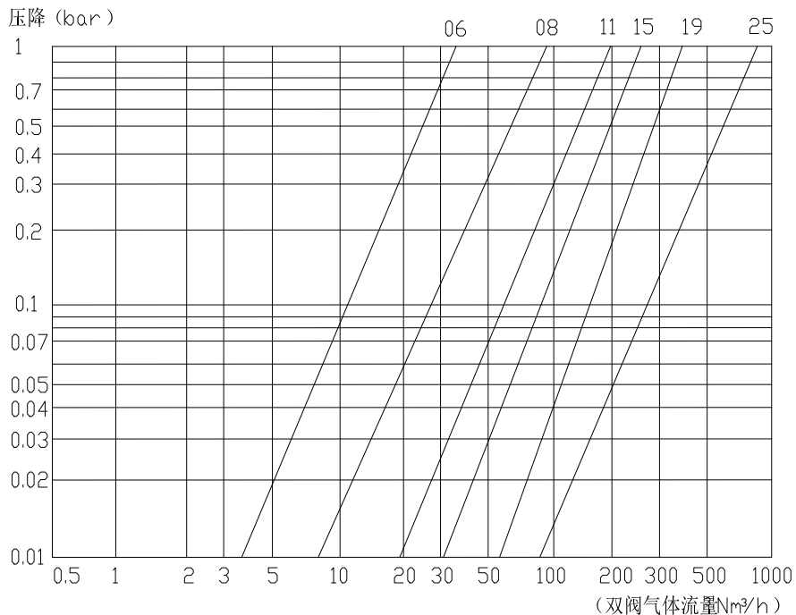
气体流量曲线图
