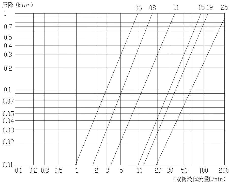
液体流量曲线图
